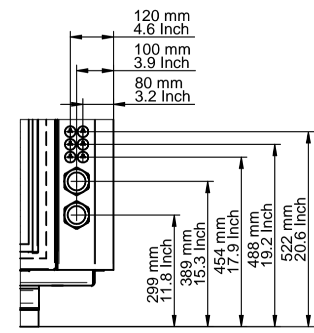
Einzelheit / Detail Y 1:10
